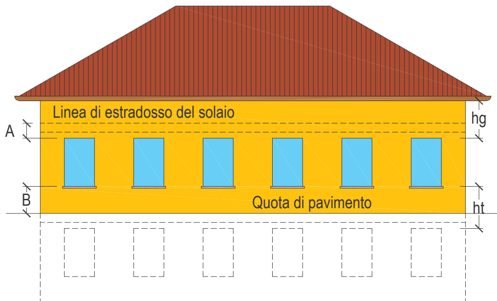
Schema di altezza di gronda (hg) riferita alla altezza teorica (ht)
